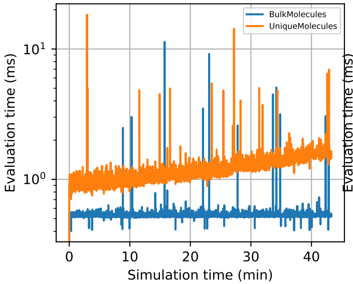
State.updateQueries
