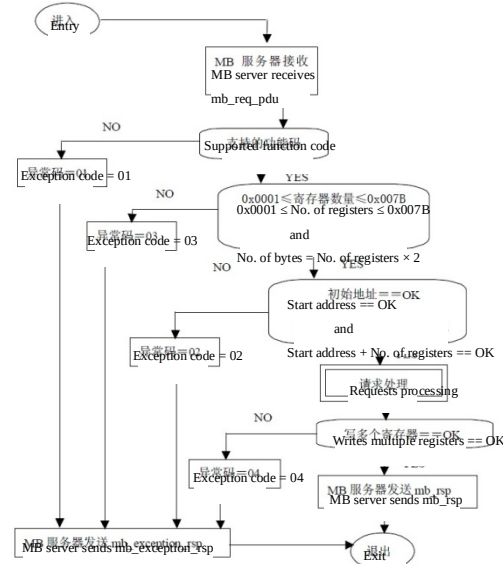
图 17 写多个寄存器的流程图 Fig. 17 Flow chart of writing multiple registers
